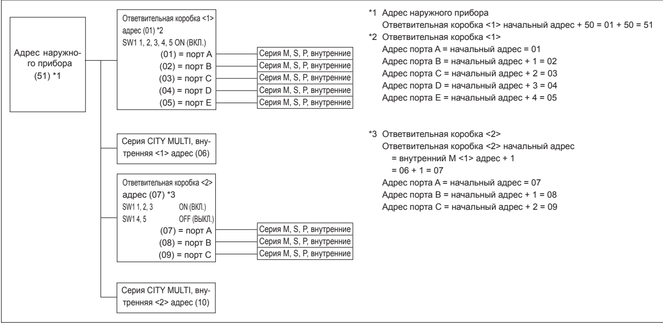
Пример 3. Наружный + ответвительная коробка <1> (серия М, S, Р, внутренние А, В, С, D, E) + ответвительная коробка <2> (серия М, S, Р, внутренние А, В, С) + серия CITY MULTI, внутренняя <1> + серия CITY MULTI, внутренняя <2>
