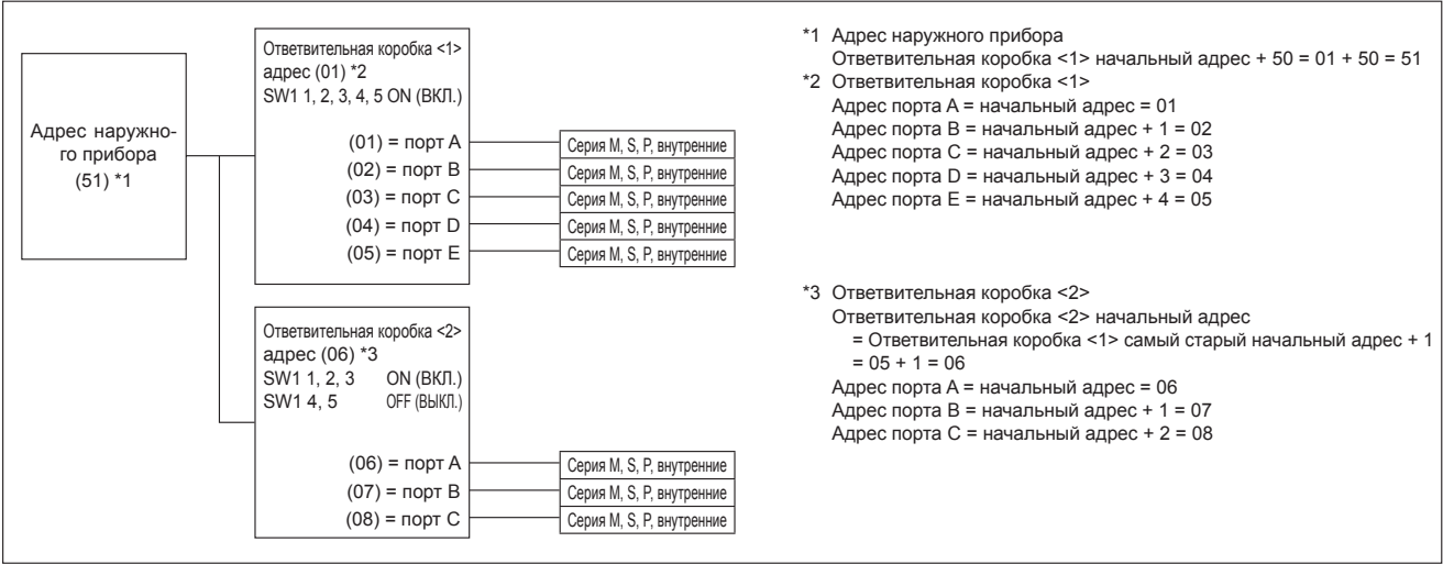
Пример 2. Наружные + ответв.коробка <1> (Серия М, S, Р, внутренние А, С, E) + ответв.коробка <2> (Серия М, S, Р, внутренние А, С, E)
