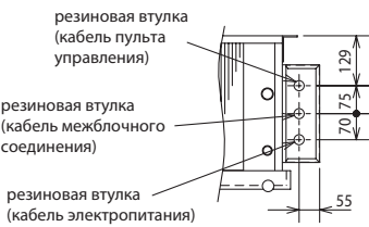
Вид спереди
